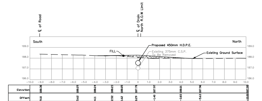
STA. 0+060
