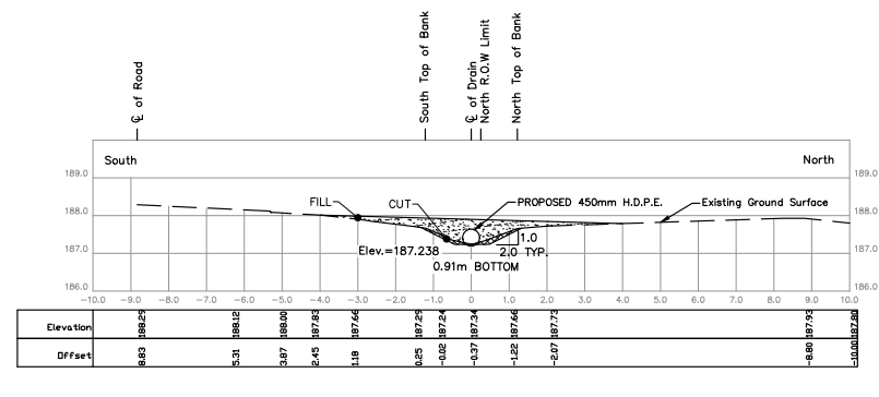
STA. 0+151 Scale = 1:100
