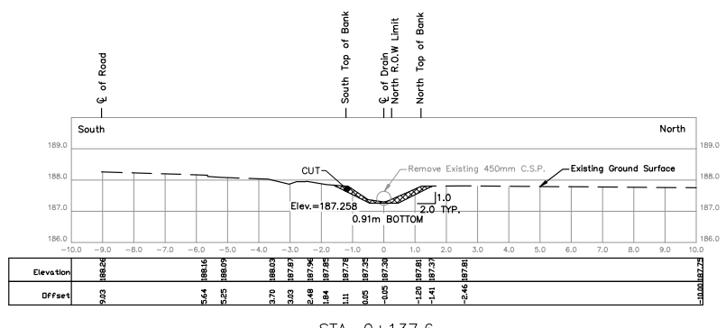
STA. 0+137.6 Scale = 1:100
