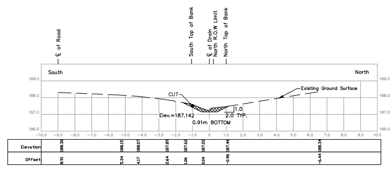
STA. 0+210 Scale = 1:100
