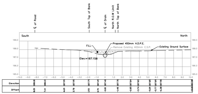
STA. 0+635.4 Scale = 1:100
