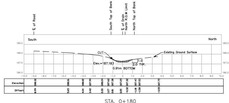
STA. 0+180 Scale = 1:100
