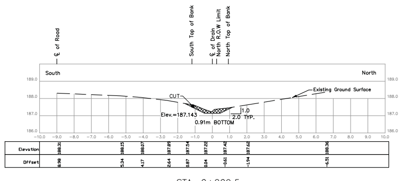
STA. 0+209.5 Scale = 1:100
