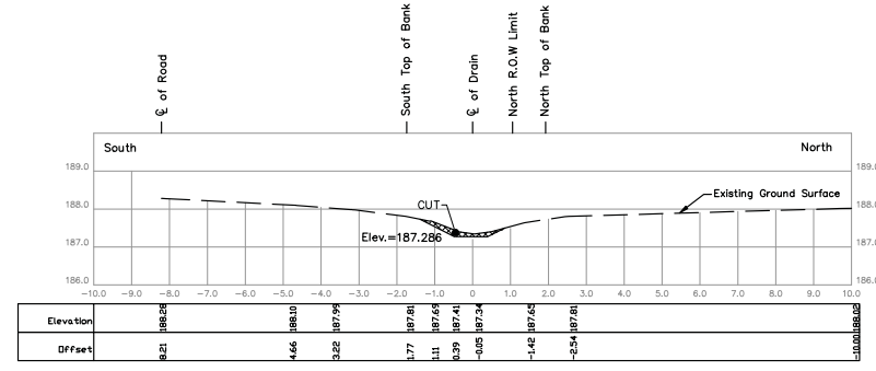
STA. 0+660 Scale = 1:100
