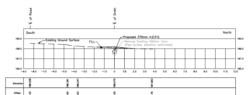
STA. 0+780.8 Scale = 1:100
