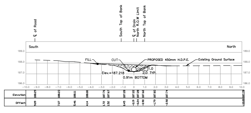
STA. 0+162.8 Scale = 1:100
