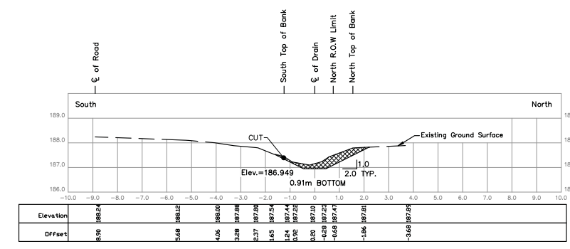
STA. 0+330 Scale = 1:100
