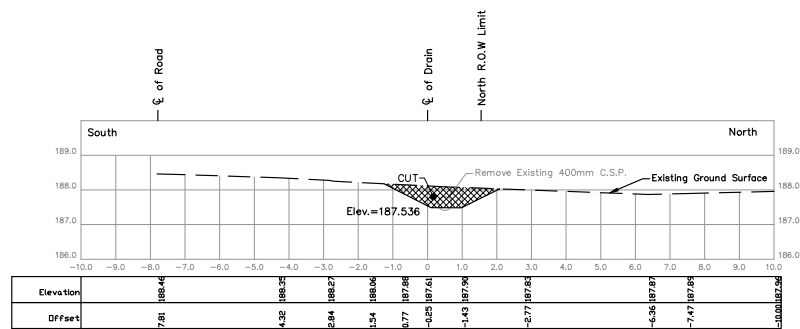
STA. 0+706.2 Scale = 1:100
