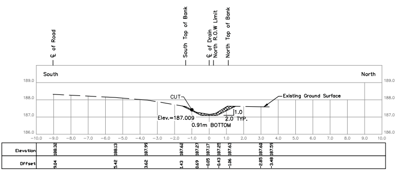
STA. 0+240 Scale = 1:100
