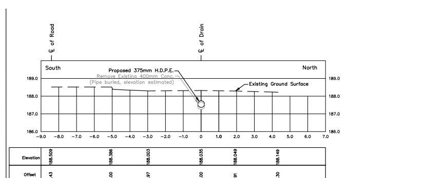
STA. 0+808.1 Scale = 1:100
