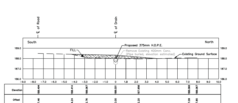
STA. 0+759.8 Scale = 1:100
