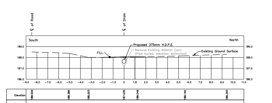
STA. 0+792.6 Scale = 1:100
