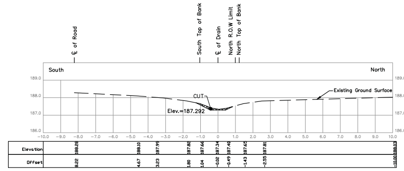
STA. 0+661.1 Scale = 1:100
