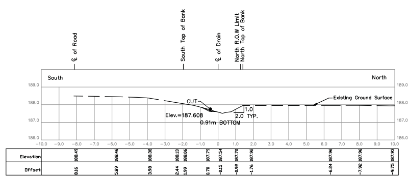
STA. 0+720 Scale = 1:100
