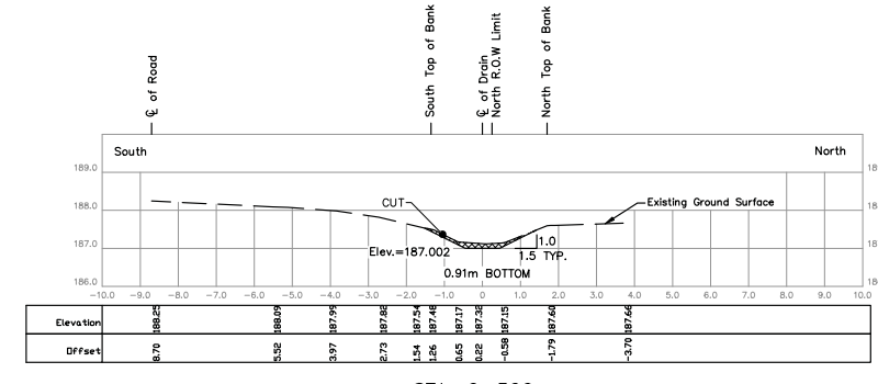
STA. 0+300 Scale = 1:100
