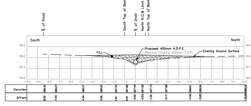
STA. 0+672.6 Scale = 1:100
