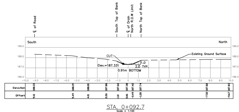
STA. 0+092.7 Scale = 1:100
