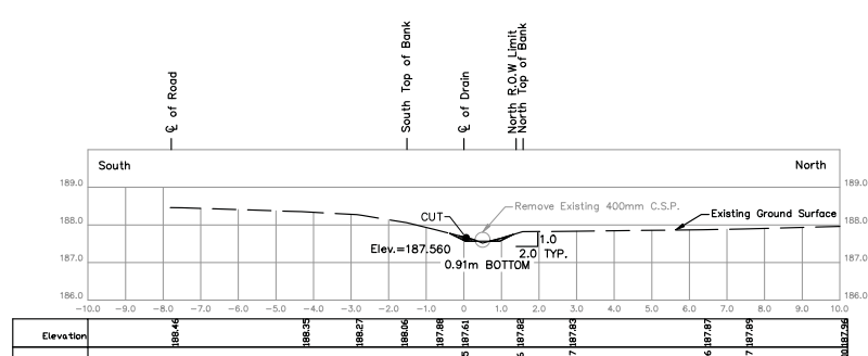
STA. 0+710.9 Scale = 1:100
