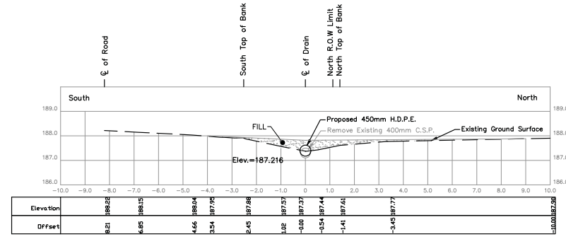
STA. 0+645.3 Scale = 1:100
