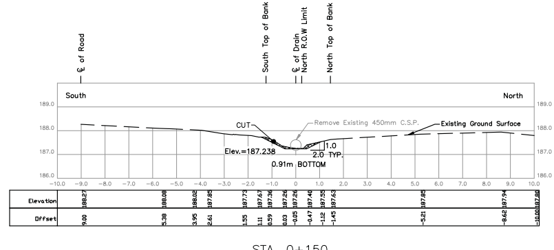
STA. 0+150 Scale = 1:100
