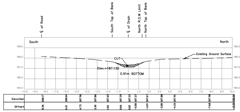
STA. 0+620.5 Scale = 1:100
