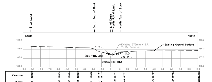
STA. 0+061.4
