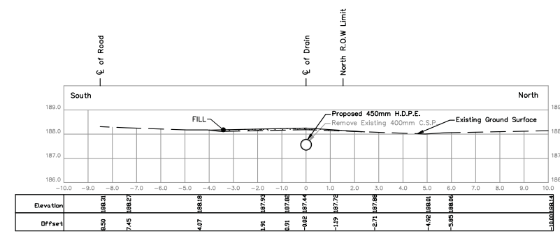
STA. 0+677.4 Scale = 1:100
