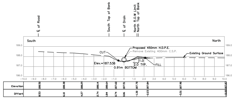
STA. 0+703.2 Scale = 1:100
