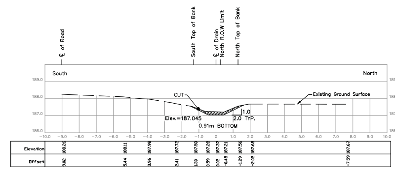
STA. 0+270 Scale = 1:100
