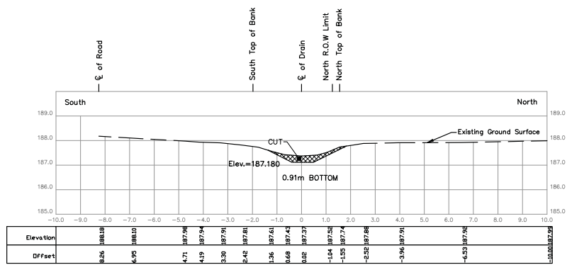
STA. 0+630 Scale = 1:100
