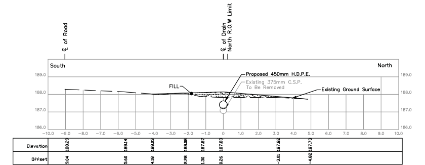
STA. 0+030
