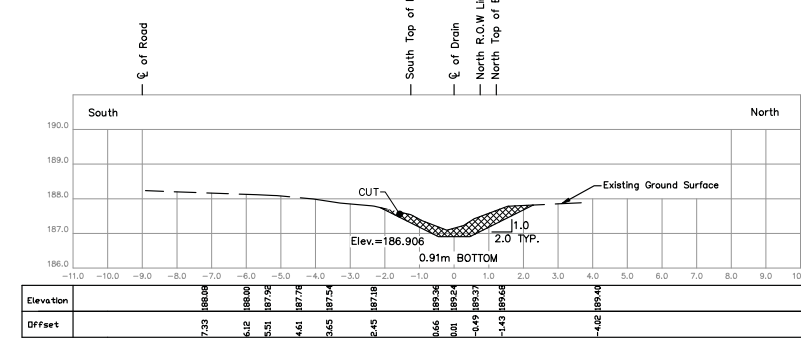
STA. 0+356.5 Scale = 1:100
