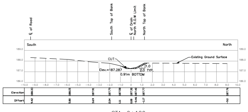
STA. 0+120 Scale = 1:100
