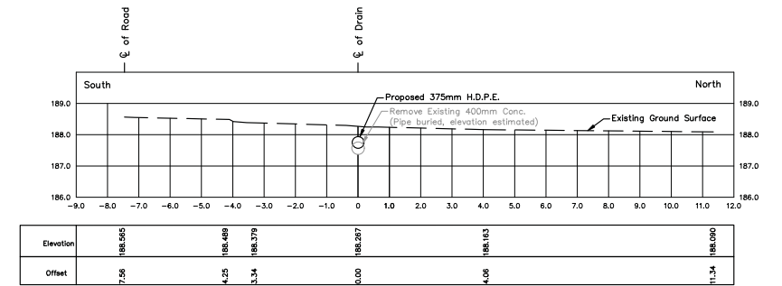
STA. 0+774.3 Scale = 1:100
