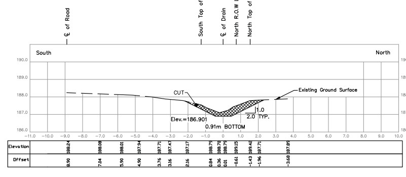
STA. 0+360 Scale = 1:100
