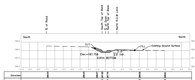
STA. 0+748.5 Scale = 1:100
