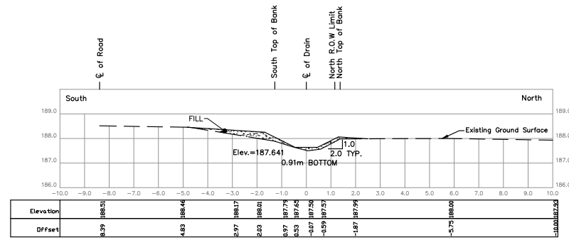
STA. 0+726.1 Scale = 1:100
