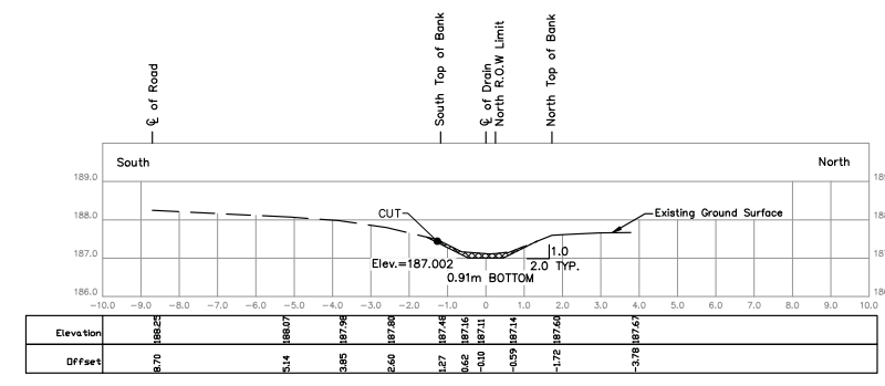
STA. 0+296.8 Scale = 1:100
