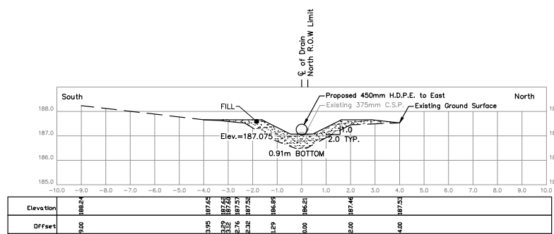
STA. 0+000
