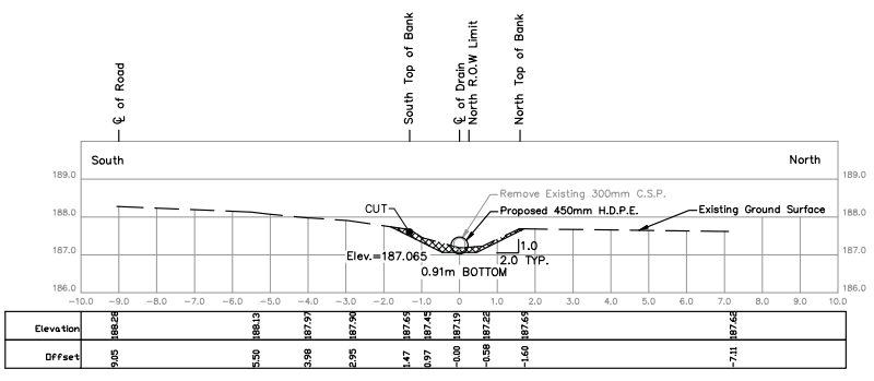
STA. 0+259.4 Scale = 1:100
