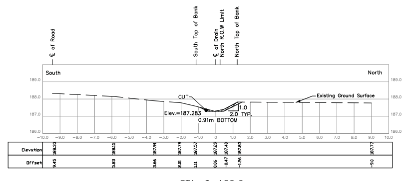
STA. 0+122.6 Scale = 1:100
