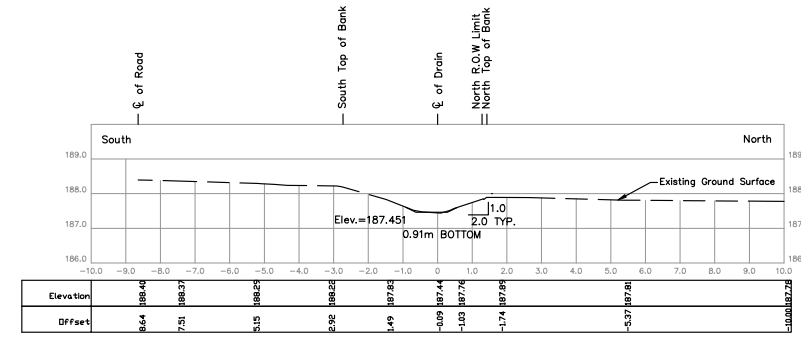
STA. 0+690 Scale = 1:100
