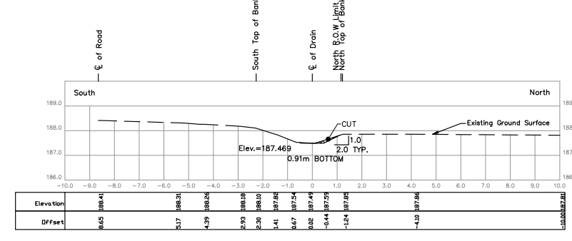
STA. 0+693.5 Scale = 1:100
