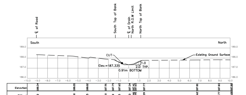
STA. 0+090
