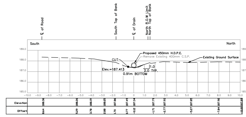
STA. 0+682.2 Scale = 1:100
